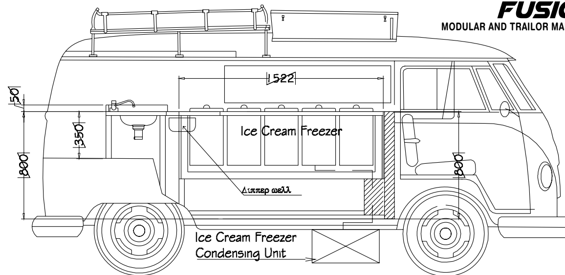
ELEVATION A
